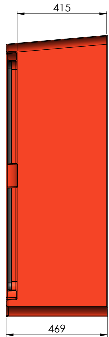
SECTION B-B SCALE 1 : 10
