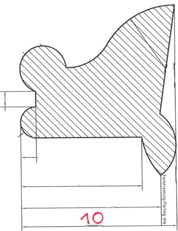
Detail X ( 10 : 1 )
